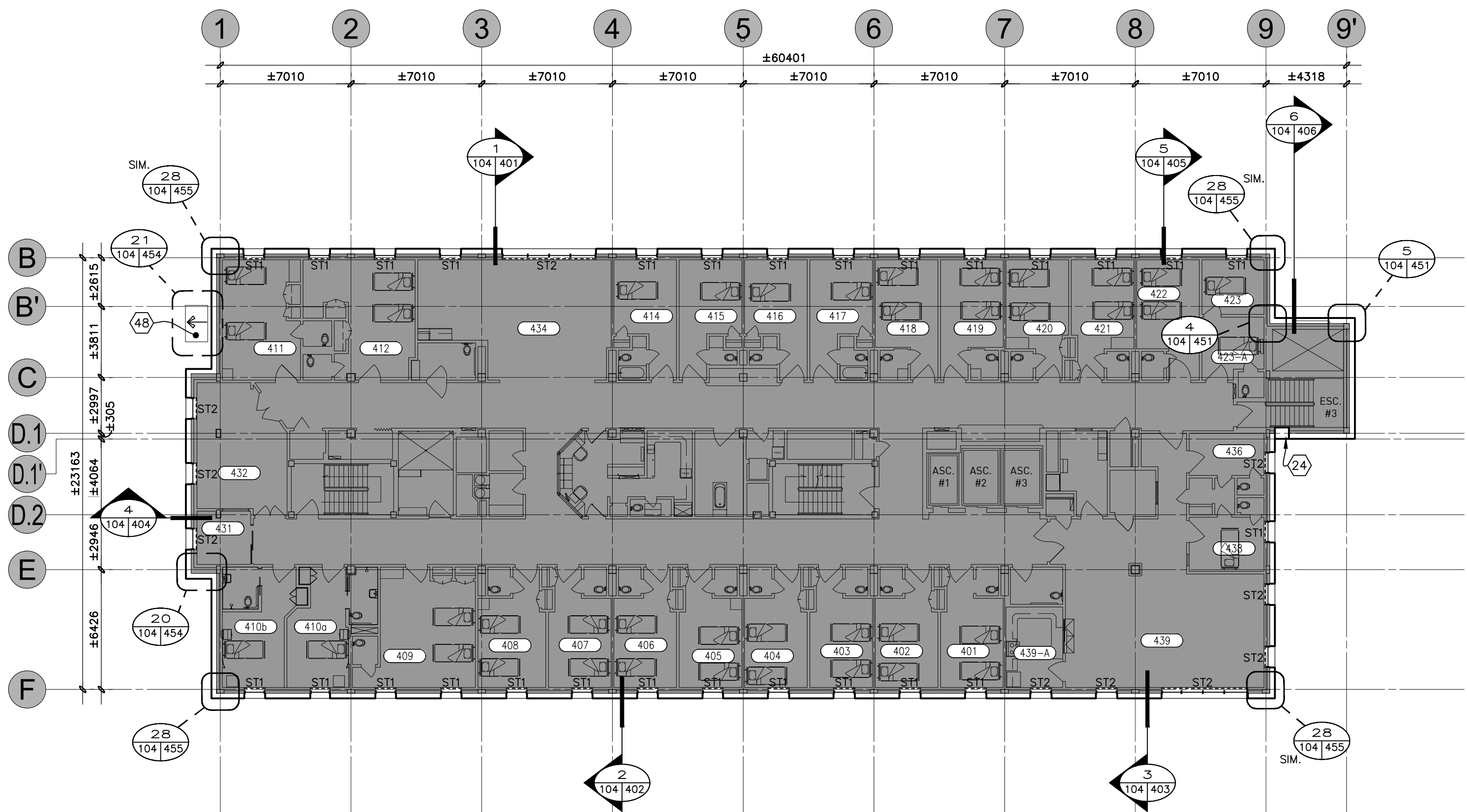
PLAN DU NIVEAU 400 - CONSTRUCTION
