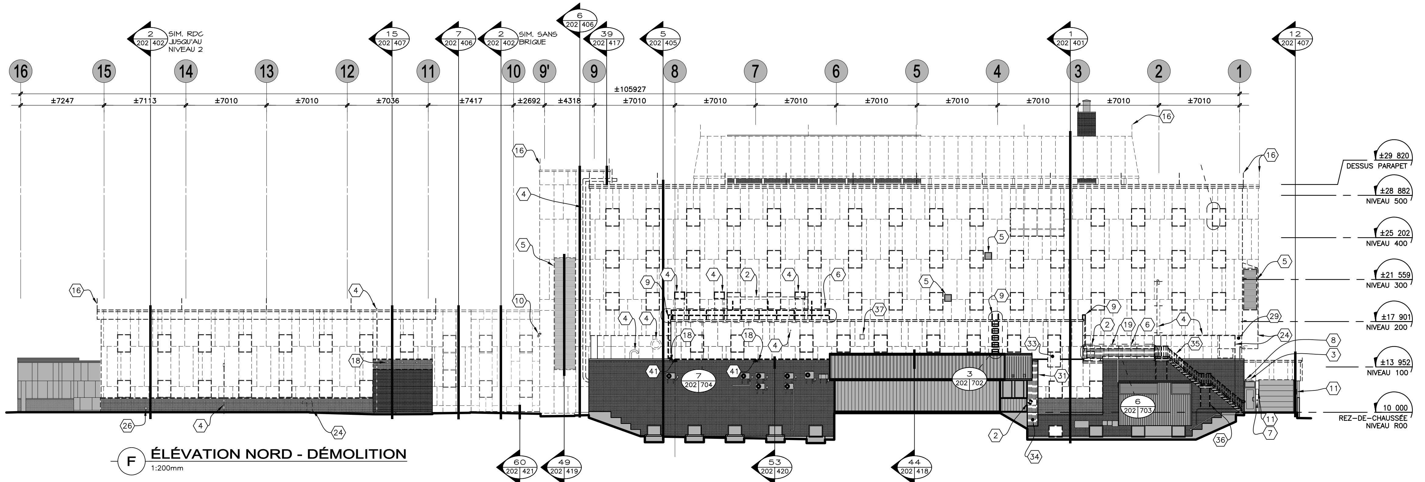
ELEVATION NORD
